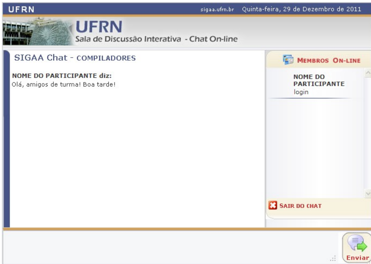
Figura 2: Mensagem
