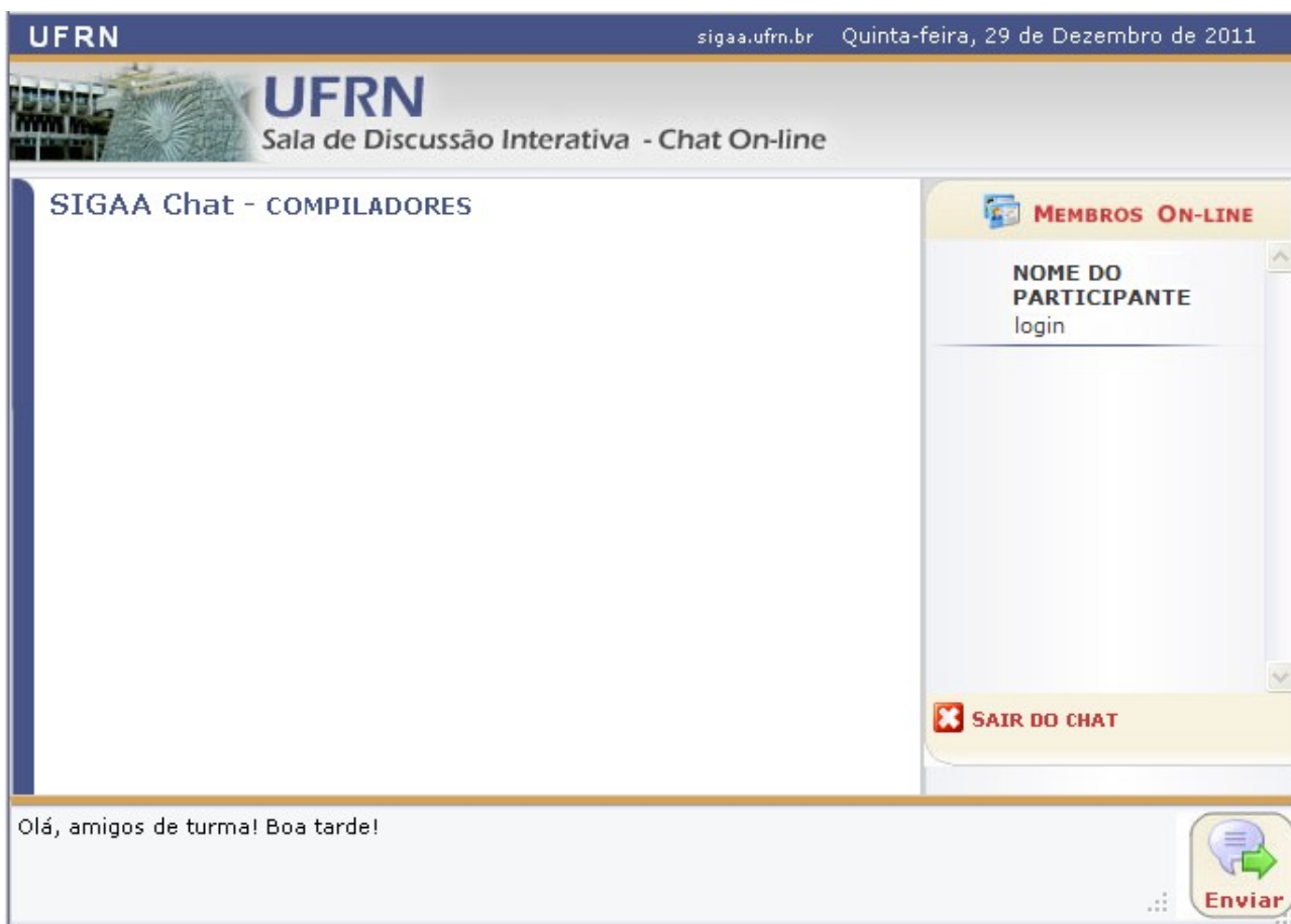
Figura 1: Chat
